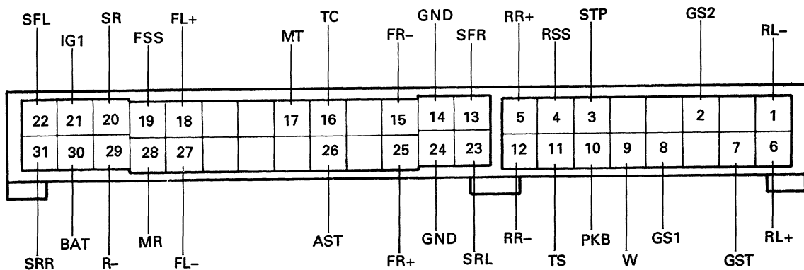
A6S ECU
